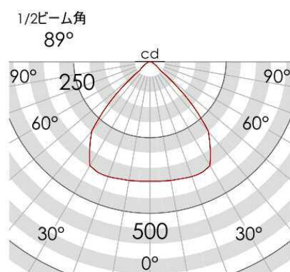
配光曲線
