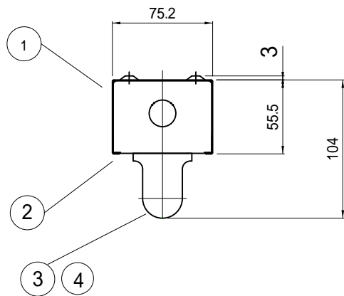
背面図
